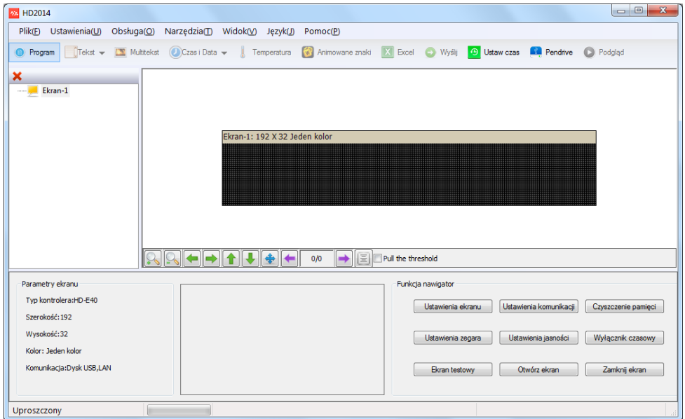
Rys. 5. Dodawanie programu.
