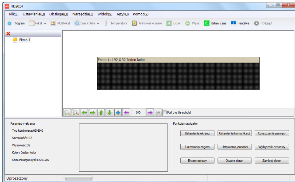
Rys. 4. Okno programu.
