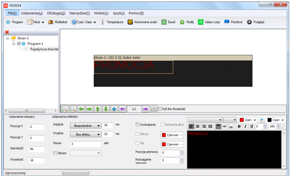
Rys. 7. Dodawanie programu.
