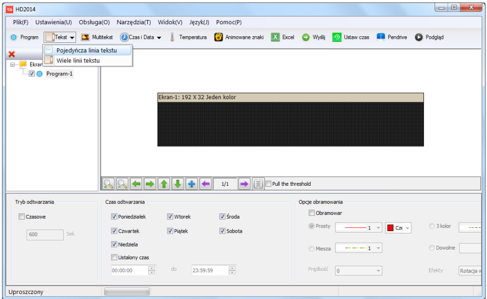
Rys. 6. Dodawanie tekstu.
